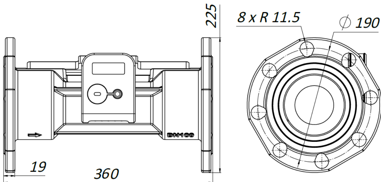
Måttskiss Qalcosonic E3 DN100 fläns
