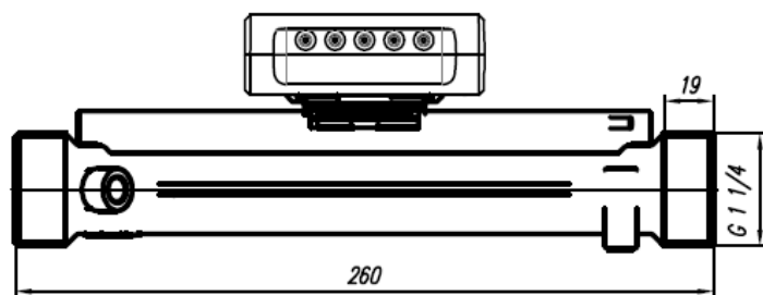
Måttskiss Qalcosonic E3 DN25 (G32 / G1¼")
