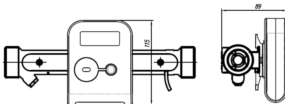
Måttskiss Qalcosonic E3 DN40 (G50 / G2")
