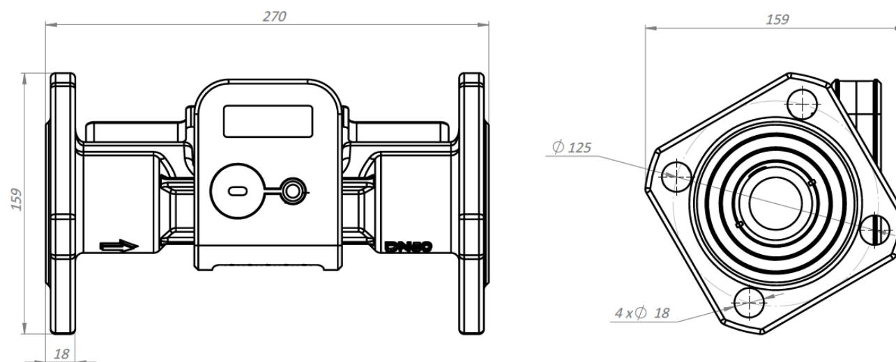
Måttskiss Qalcosonic E3 DN50 fläns
