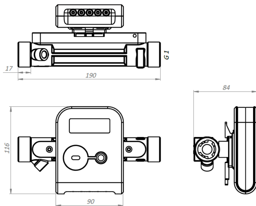
Måttskiss Qalcosonic E3 DN20 (G25 / G1") 190mm
